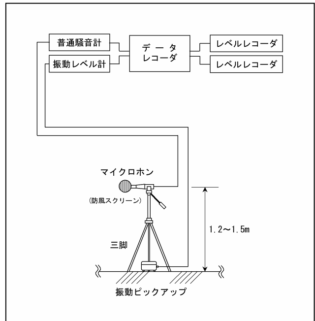
図-1 騒音・振動計測概念図
